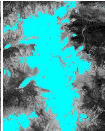
Figura 9: NDSI (Reflectancia)
