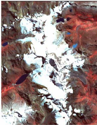
Figura 7: RGB 321 – ASTER
