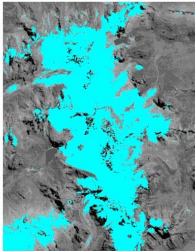
Figura 8: NDSI (Radiancia)
