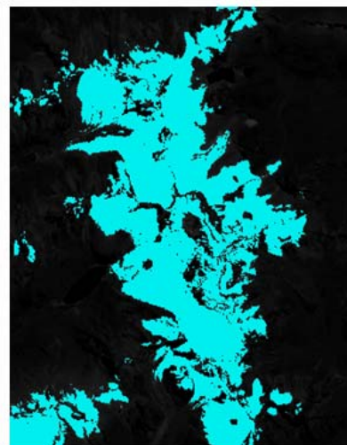
Figura 6: Ratio (Reflectancia)
