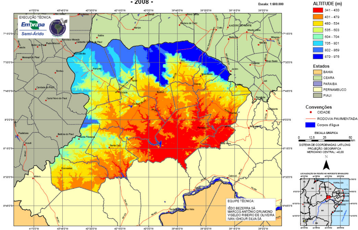
Figura 2. Modelo digital de elevação da região do Araripe pernambucano.
