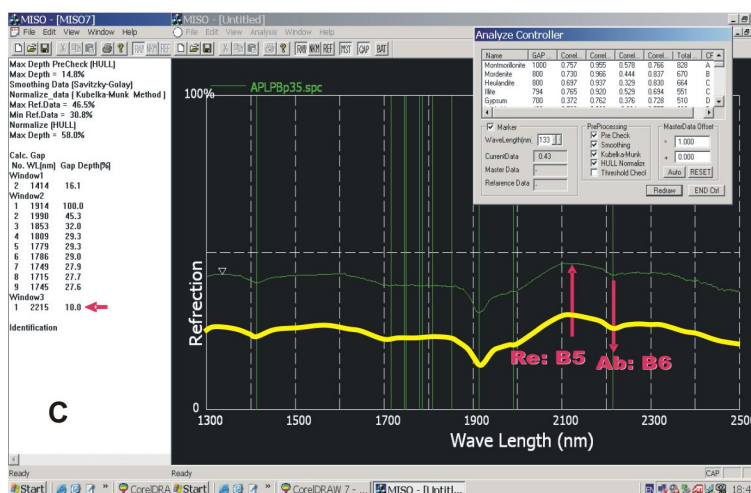
Figura 3 - Assinaturas espectrais obtidas no espectrorradiômetro POSAM. A: conjunto dos espectros medidos; B: espectro de rocha básica, reflete na banda 4 e absorve na banda 7; C: espectro de rocha ácida a intermediária, reflete na banda 5 e absorve na banda 6; relativos aos comprimentos de onda das bandas do ASTER (SWIR).
