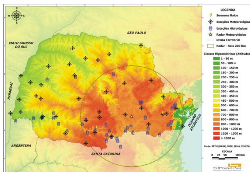
Figura 2. Estações meteorológicas telemétricas do Instituto Tecnológico SIMEPAR
